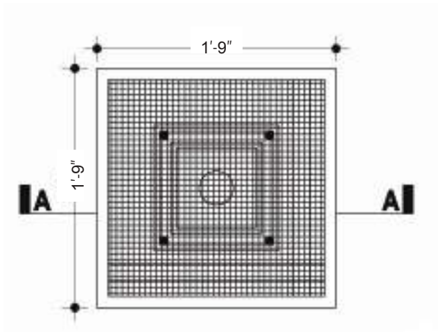
Plan of FC pocket footing F1
